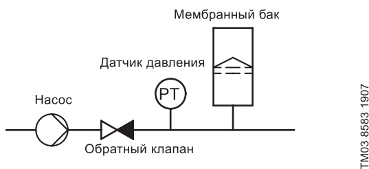
Рис. 24 Расположение обратного клапана и датчика давления в системе, имеющей подпор на входе
