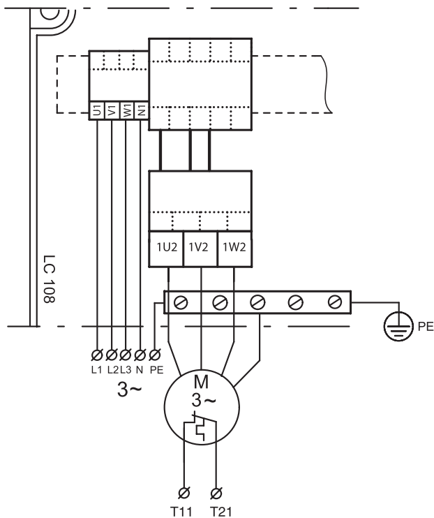
3~ DOL
