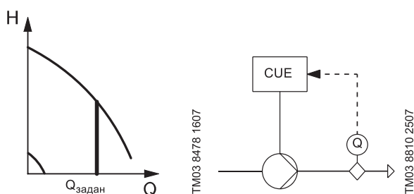
Рис. 11 Постоянный расход
