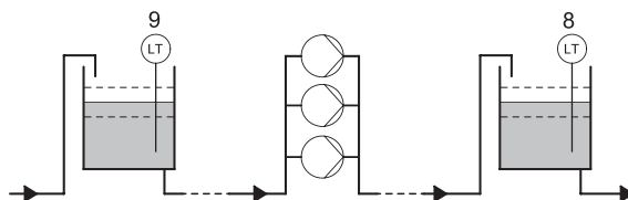
Рис. 33 Контроль уровня
