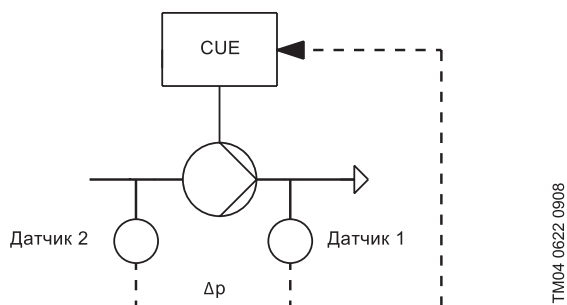
Рис. 32 Перепад давления от двух датчиков
