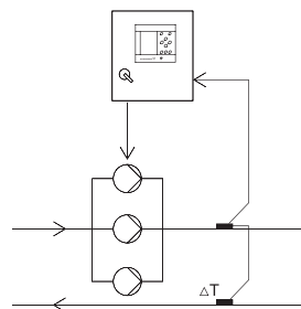
Рис. 27 Перепад температур
